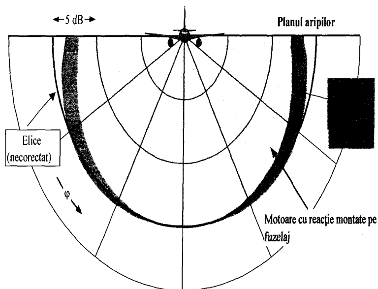
Figura 2.7.n: Direcționalitatea laterală a efectelor amplasării
