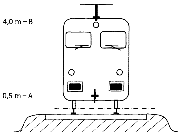
Figura [2.3.a]: Amplasarea surselor de zgomot echivalente
