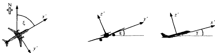
Figura 2.7.c: Sistemul de coordonate fixe al aeronavei (x',y',z')
