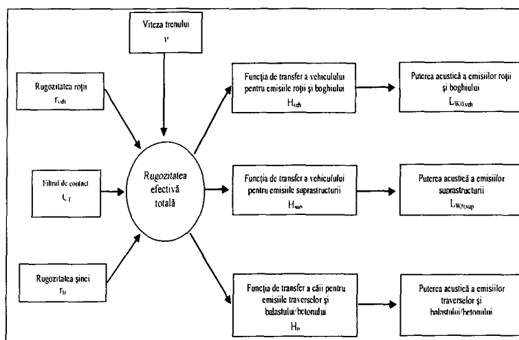
Figura [2.3.c]: Schema utilizării diferitelor definiții ale rugozității și funcțiilor de transfer.
